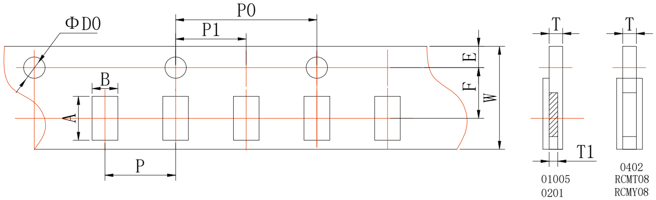
单位 unit: mm
